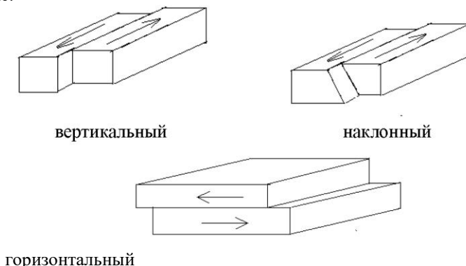
Рис. 31. Типы сдвигов
