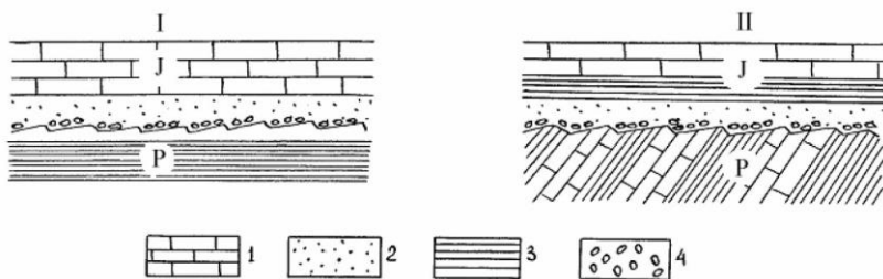
Рис. 11. Типы несогласий I - параллельное, II - угловое 1 - известняк, 2 - песок, 3 - аргиллит, 4 - конгломерат
