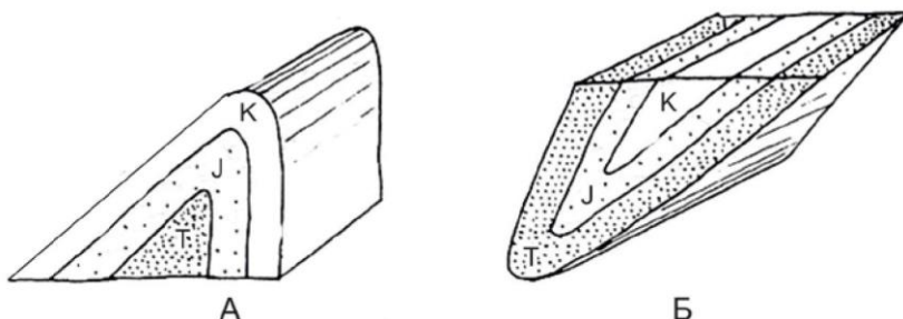
Рис. 20. Антиклинальная (А) и синклиналиная (Б) складки горизонтальную плоскость; изменяется от 0 до 90°.
