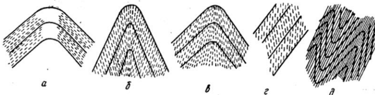
Рис. 34. Разновидности кливажа
