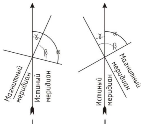
Рис. 17. Схема, поясняющая введение поправки на магнитное склонение I - в случае восточного, II - в случае западного склонения; а - истинный азимут; в - магнитный азимут; γ - магнитное склонение
