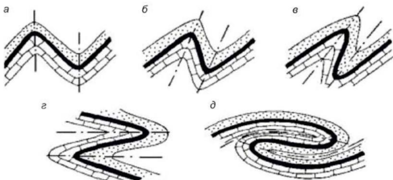
Рис. 23. Классификация складок по положению осевой поверхности и падению крыльев складки
