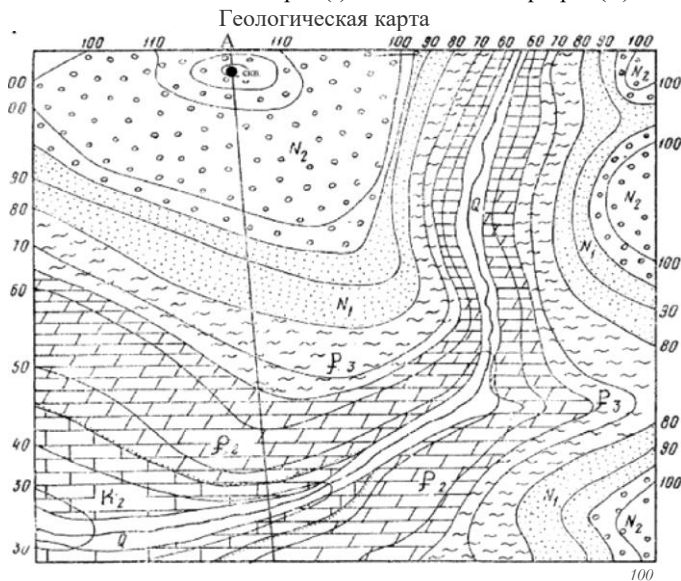
Рис. 12. Геологическая карта (I) и геологический разрез (II)
