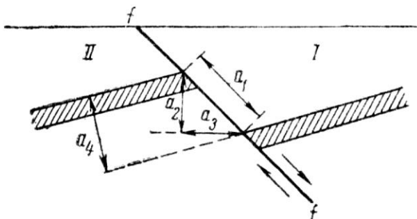
Рис. 28. Элементы разрывных нарушений I, II - крылья; f-f - сместитель; амплитуда: a_1 - по сместителю, a_2 - вертикальная, a_3 - горизонтальная, a_4 - стратиграфическая; a - угол падения сместителя
