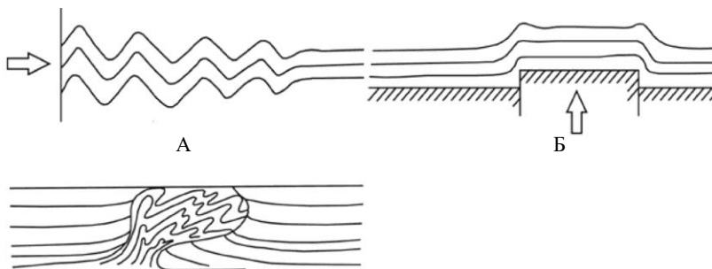
Рис. 21. Генетические типы складчатости А - продольного изгиба, Б - поперечного изгиба, В - нагнетания (пластического течения). Стрелками показано направление движения масс
