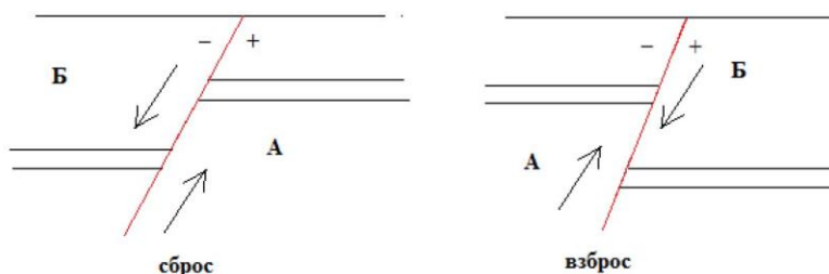
Рис. 29. Схема строения сброса и взброса
