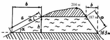
Рис. 10. Мощность слоя и ее определение
