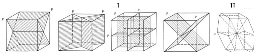
Рис. 2. Элементы симметрии
