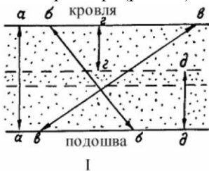
Рис. 10. Мощность слоя и ее определение
