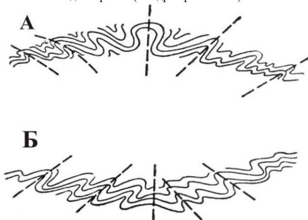
Рис. 27. Схема антиклинория (А) и синклиория (Б) в вертикальном поперечном разрезе Крупные складчатые структуры на платформах в виде обширных
