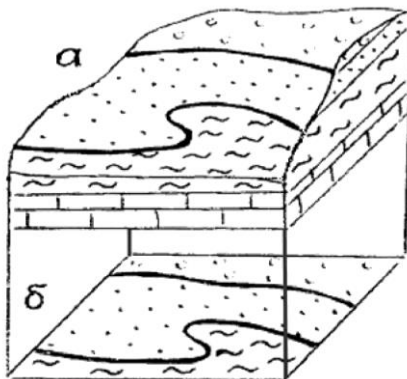
Рис. 9. Линии выходов поверхностей наслонения (утолщенные линии) на блок-диаграмме (а) и на плане (б)
