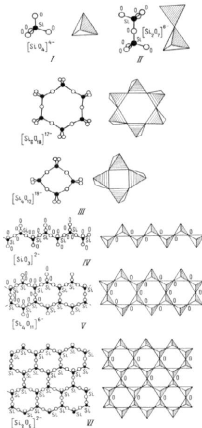
Рис. 5. Структура силикатов
